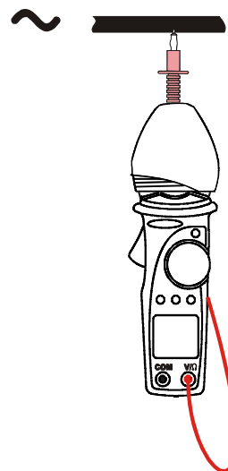
Fig. 17: busca fases con capuchón de goma
