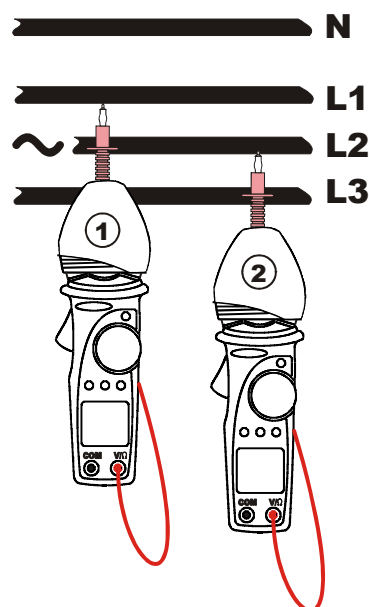
Fig. 13: detección de la secuencia de las fases con capuchón de goma
