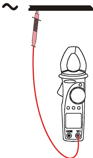
Fig. 16: busca fases
