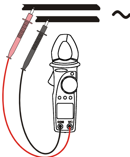
Fig. 6: medida de frecuencia con puntas de pruebas
