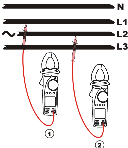
Fig. 12: detección de la secuencia de fases
